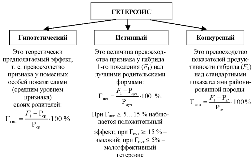
Рис. 13. Типы гетерозиса
